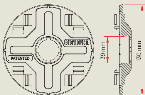
Versione autolivellante per supporti PR e SE Tilting version for PR and SE supports
