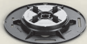
Supporto New Maxi NM 0 da H 15 mm
